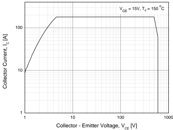
Fig. 15 RBSOA
