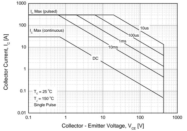
Fig. 14 SOA
