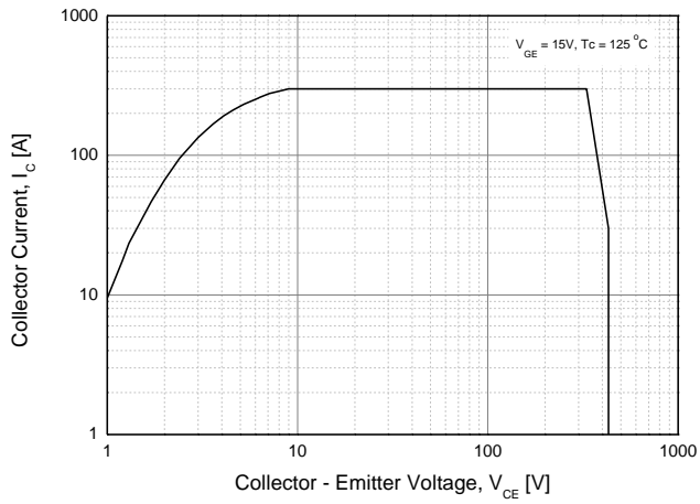
Fig. 15 RBSOA
