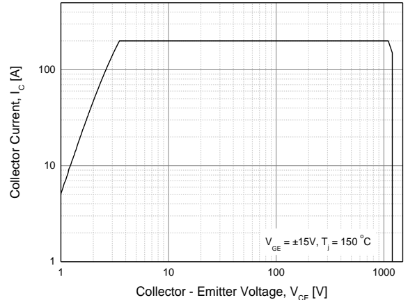
Fig. 12 RBSOA
